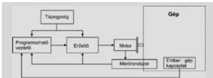
1. ábra Egyszerű mozgásvezérlő rendszer blokkvázlata
